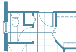
Master Bath Door Option
